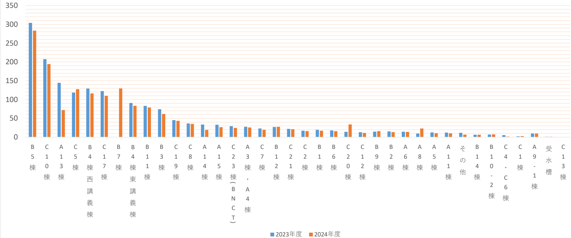
中百舌鳥キャンパス棟別使用量(MWh/11月)
